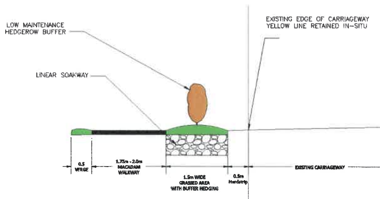
Askeaton Slí na Sláinte Detail
