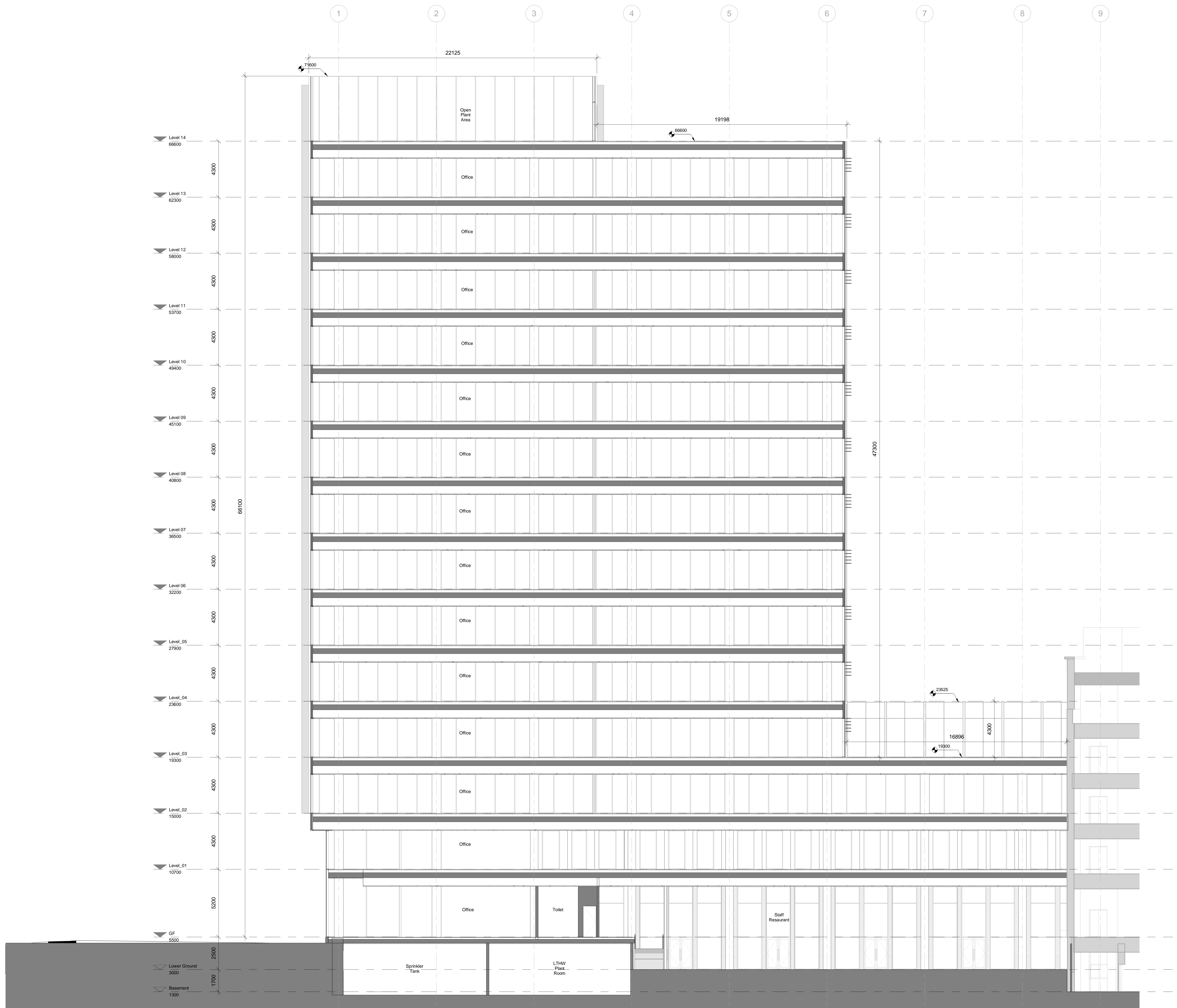
1 Section A-A SCALE: 1 : 100
